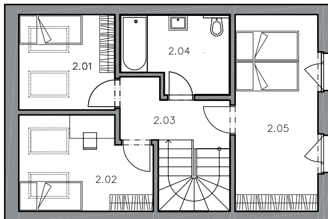
PŮDORYS 2.N.P.
