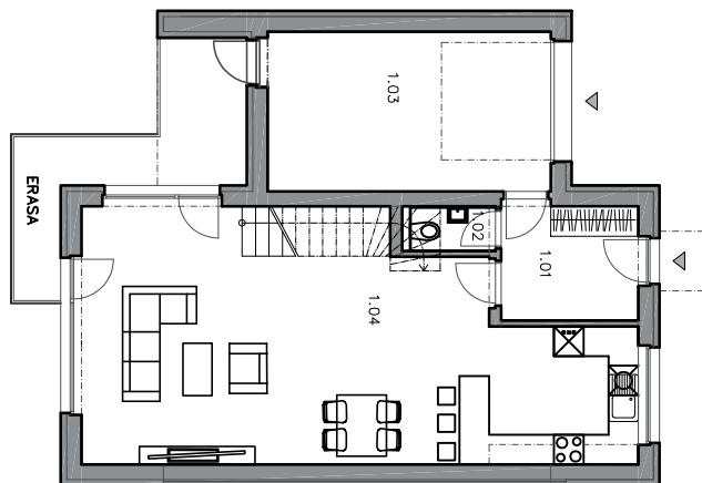
PŮDORYS 1.N.P.
