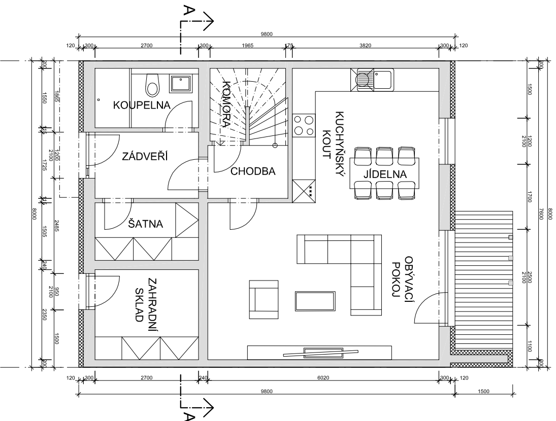
PŮDORYS 1.NP
