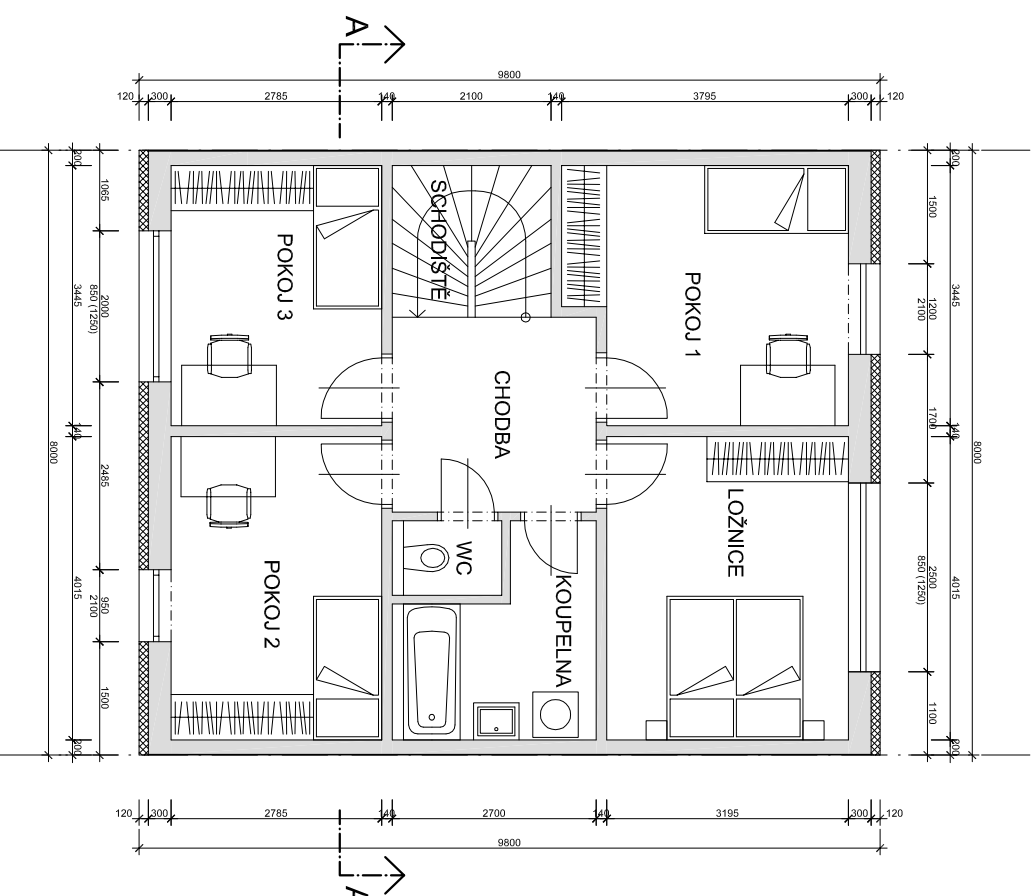
PŮDORYS 2.NP
