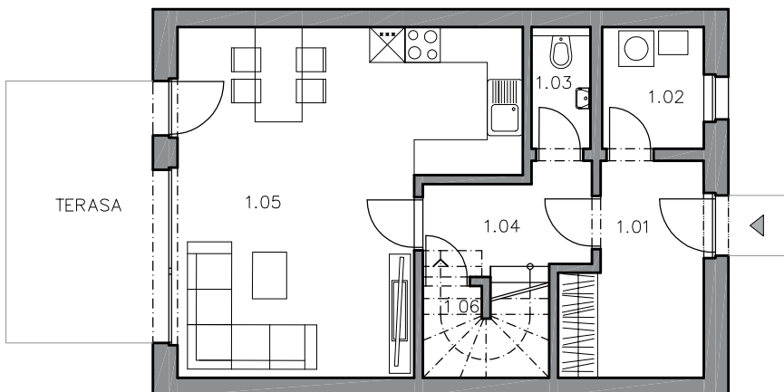
PŮDORYS 1.N.P.
