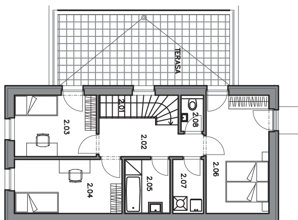
PŮDORYS 2.N.P.
