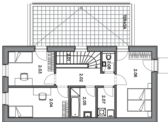
PŮDORYS 2.N.P.
