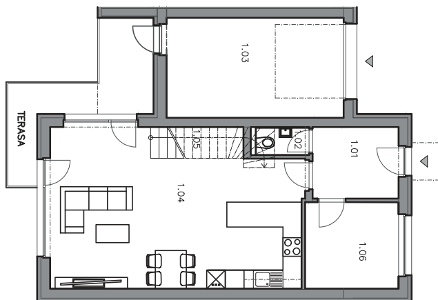
PŮDORYS 1.N.P.
