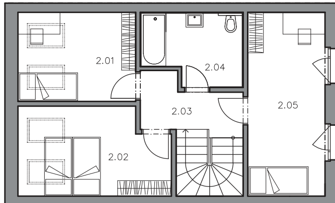
PŮDORYS 2.N.P.
