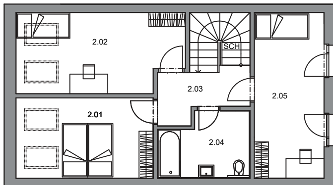
PŮDORYS 2.N.P.
