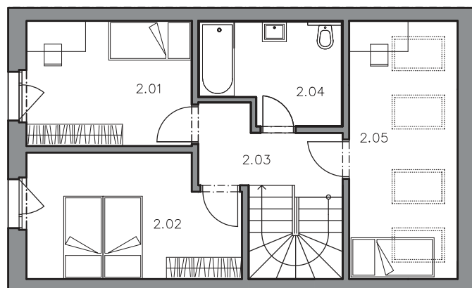
PŮDORYS 2.N.P.
