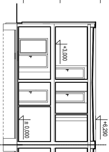
ŘEZ A-A
