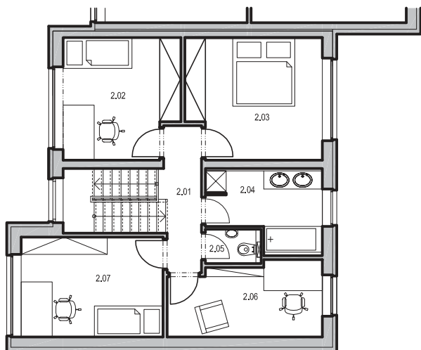
PŮDORYS 2.N.P.
