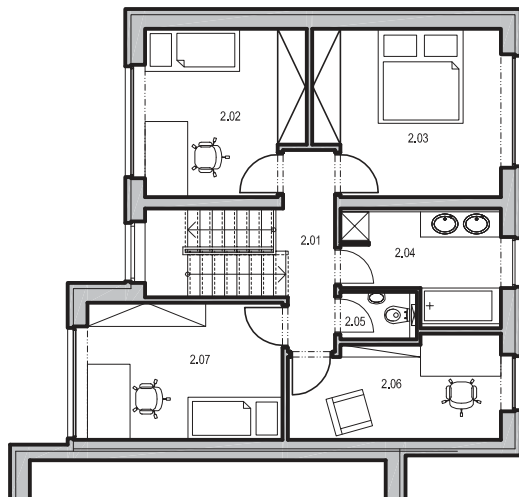
PŮDORYS 2.N.P.
