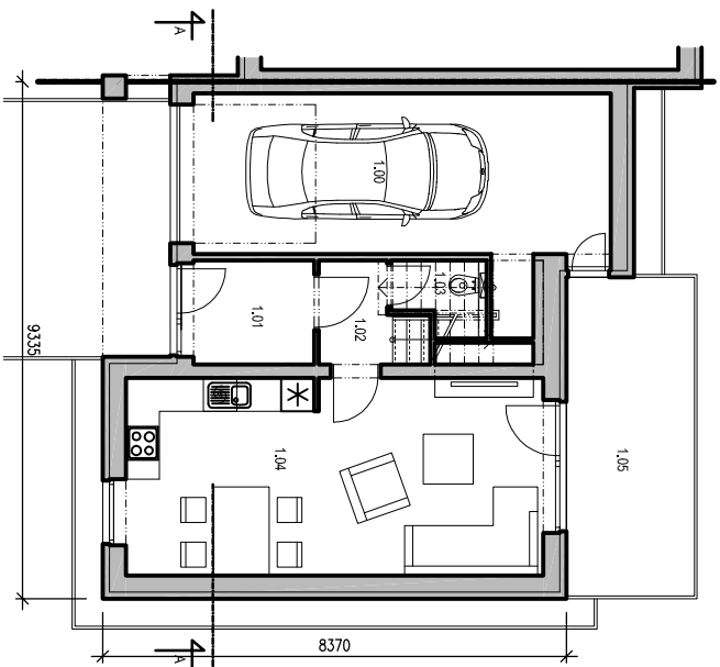
1. NADZEMNÍ PODLAŽÍ
