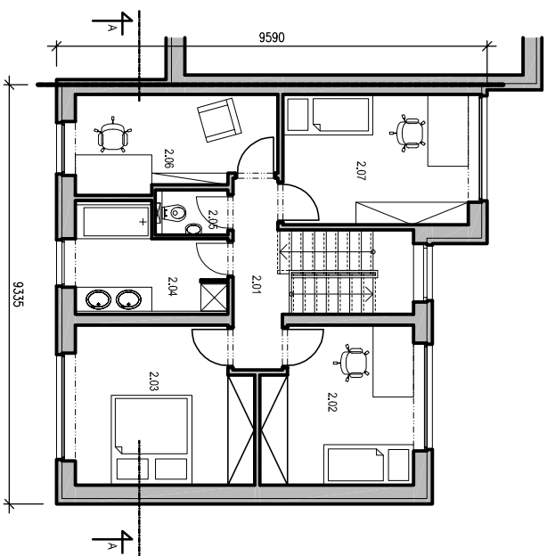
2. NADZEMNÍ PODLAŽÍ
