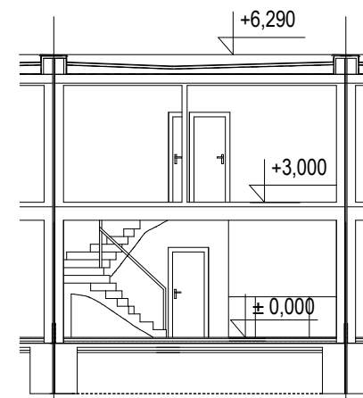
ŘEZ A-A
