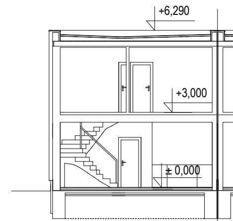
ŘEZ A-A
