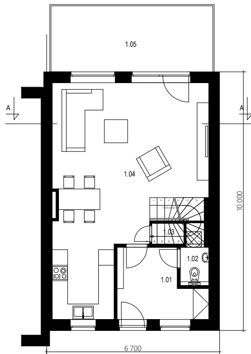
1.NADZEMNÍ PODLAŽÍ
