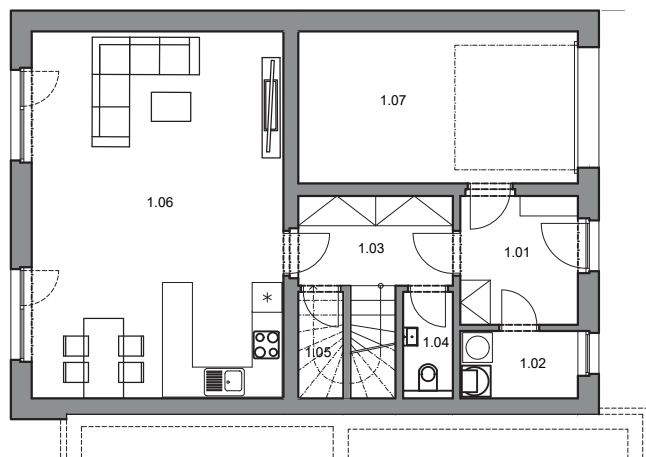
PŮDORYS 1.N.P.
